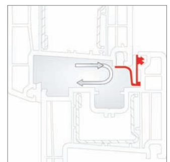
La creșterea presiunii vântului sistemul REHAU AirComfort se închide automat, pe baza principiului lui Bernoulli.
