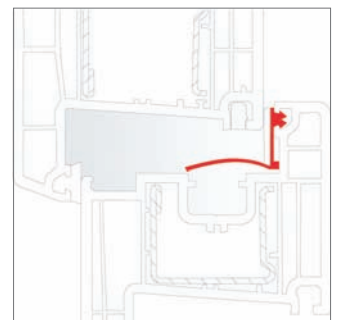
Poziția de aerisire în caz de presiune normală a aerului.
